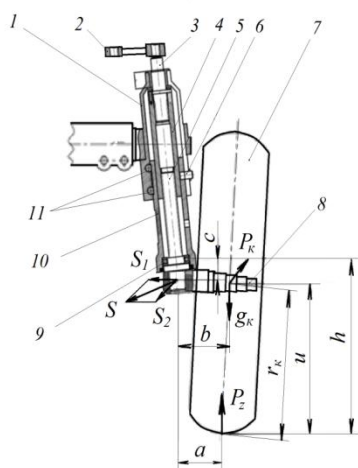
Рисунок 1 – Силы, действующие на шкворень поворотной цапфы при встрече передних колес с непреодолимым препятствием
