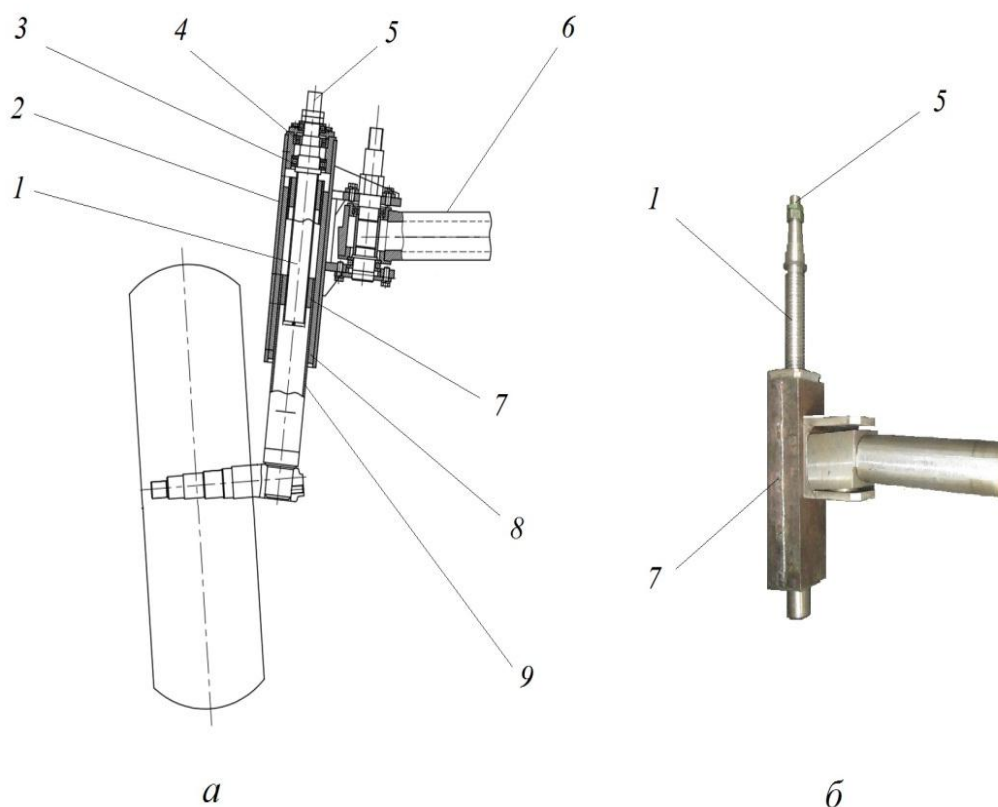
Рисунок 1 – Винтовой механизм регулировки клиренса переднего моста в схеме (а) и в натуре (б)
