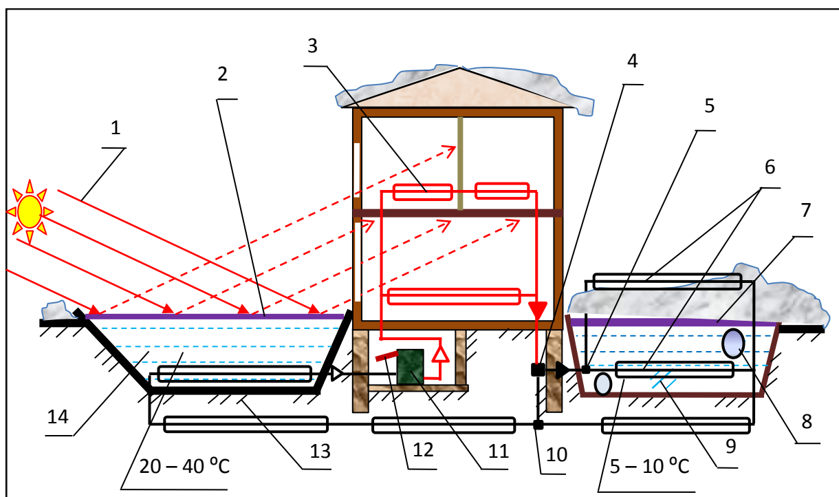
1 – солнечное излучение; 2, 7 – теплоизоляционное покрытие; 3 – конденсатор теплового насоса; 4 – дроссель; 5, 10 – регулятор потока хладагента; 6 – испаритель теплового насоса; 8 – воздуховод; 9 – котлован с талой водой; 11 – хладомёт (двигатель Стирлинга с компрессором); 12 – тепловая гравитационная труба (термосифон); 13 – грунт; 14 – солнечный соляной пруд
