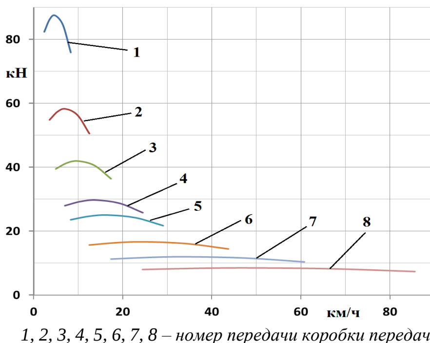
Рисунок 5 – Тягово-скоростная характеристика автомобиля КрАЗ-6322
