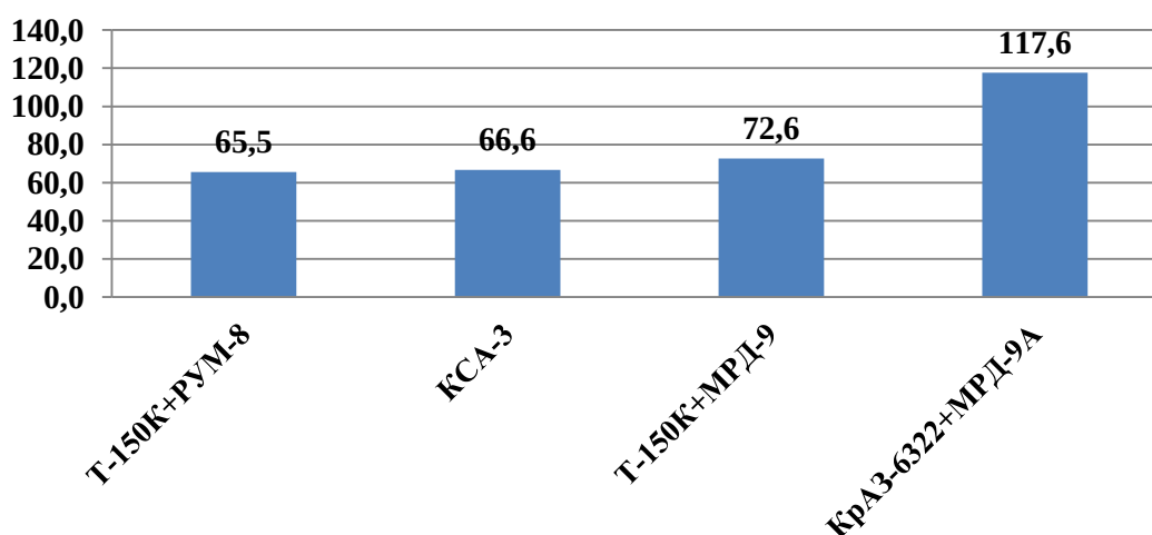
Рисунок 7 – Сменная производительность МТА по прямоточной схеме внесения минеральных гранулированных удобрений
