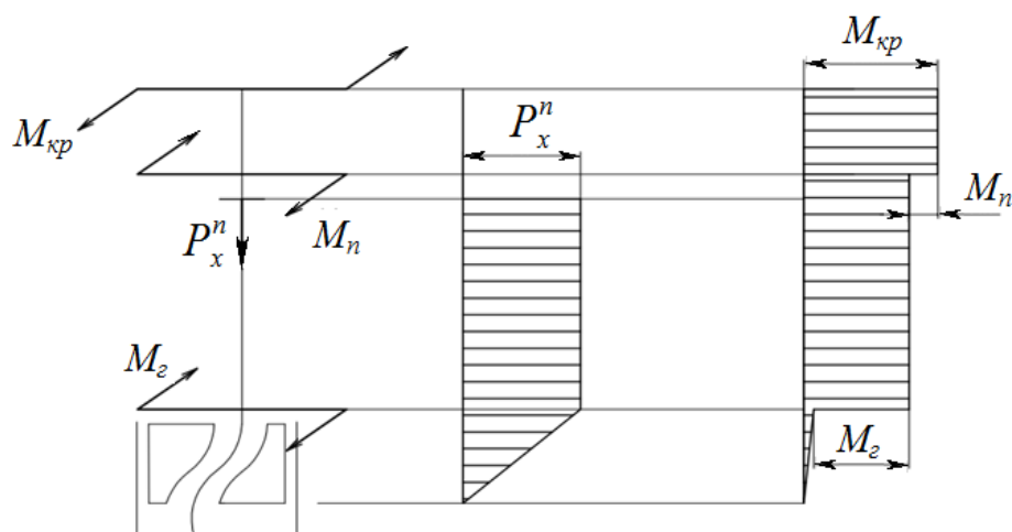
Рисунок 2 – Эпюры продольных сил и крутящих моментов, действующих на винт при подъеме балки переднего моста
