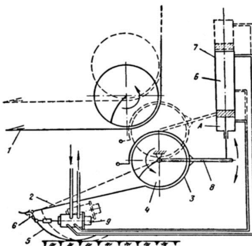
Рисунок 19 – Схема устройства для установки положения стриппера в зависимости от высоты установки хедера
