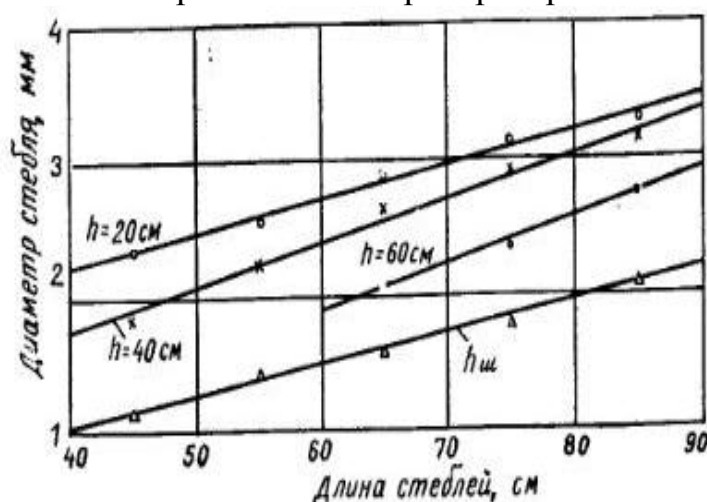
Рисунок 2 – Изменение диаметра стебля по его высоте для стеблей различной длины
