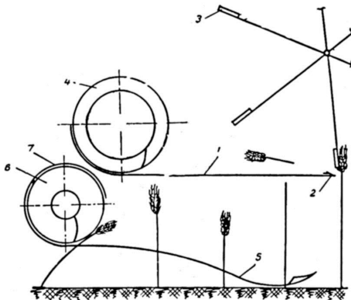
Рисунок 1 – Колосоуборочная машина в продольном разрезе
