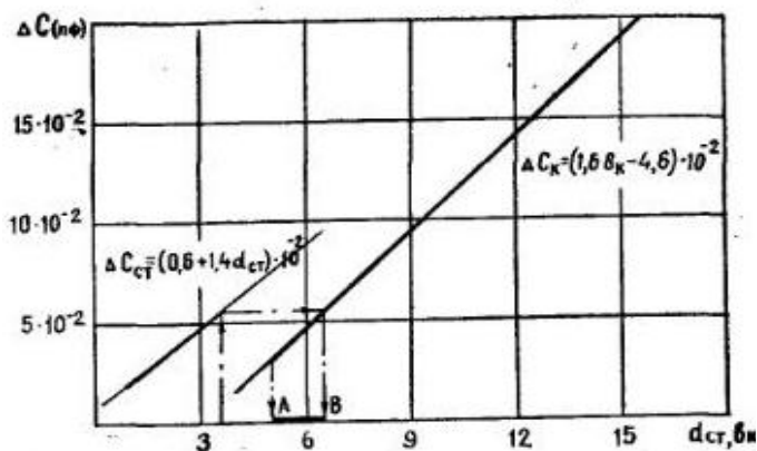
Рисунок 17 – Изменение емкости конденсатора от диаметра стеблей и ширины колосьев
