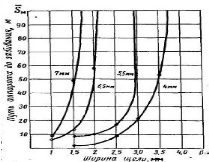
Рисунок 3 – Зависимость пути забивания рабочей щели стриппера от ее ширины при различных размерах пластиковой кромки
