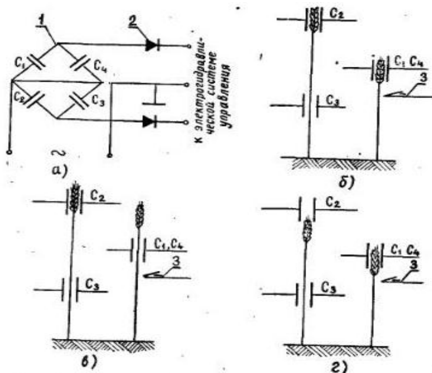
Рисунок 18 – Схема работы емкостного датчика высоты среза
