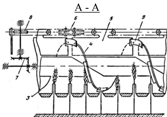
Рисунок 8 – Устройство для предотвращения выбрасывания срезанных колосьев из стриппера
