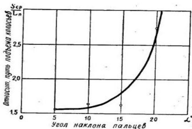
Рисунок 6 – Относительный путь транспортирования при различных углах наклона вычесывающих пальцев стриппера
