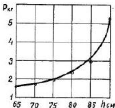
Рисунок 12 – Усилия отрыва колоса от стеблей в зависимости от его длины
