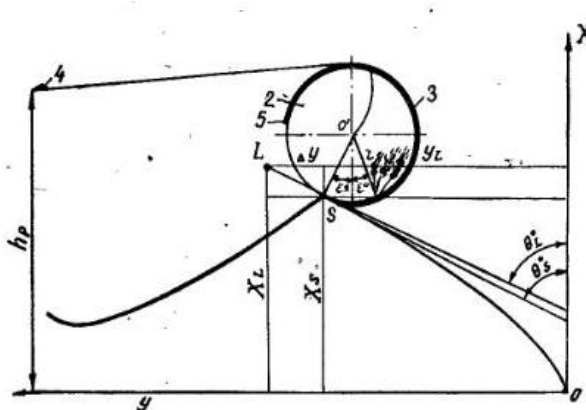
Рисунок 5 – К обоснованию длины зоны резания стриппера
