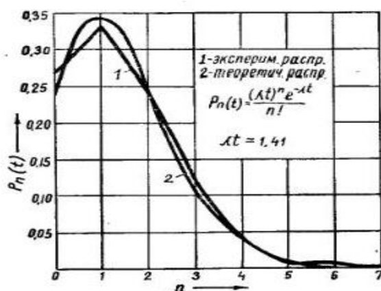
Рисунок 4 – Распределение потока требований в щели стриппера
