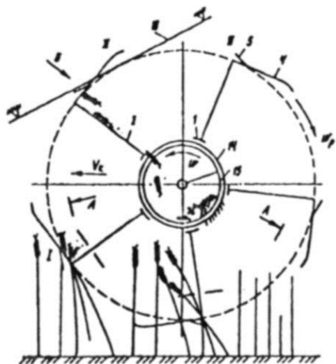
Рисунок 9 – Очесывающий аппарат для уборки зерновых культур на корню
