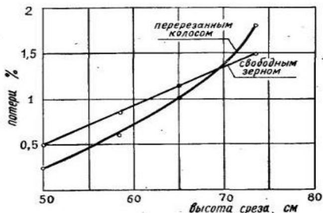
Рисунок 16 – Потери осыпавшегося зерна от перерезанных колосьев в зависимости от высоты установки режущего аппарата хедера-стриппера
