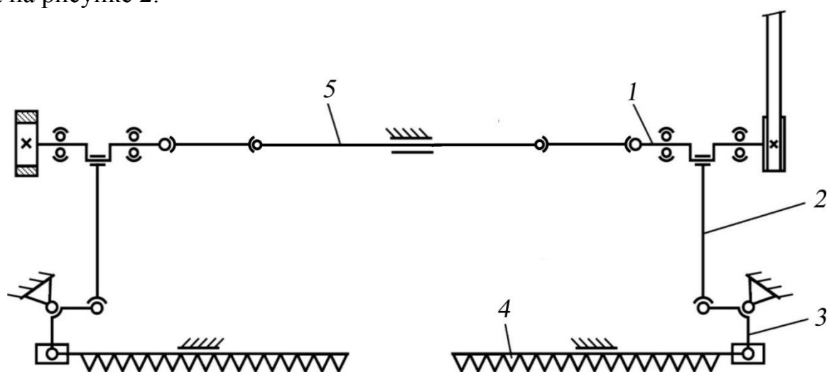
Рисунок 2 – Схема привода двухножевого режущего аппарата с кривошипно-коромысловыми механизмами
