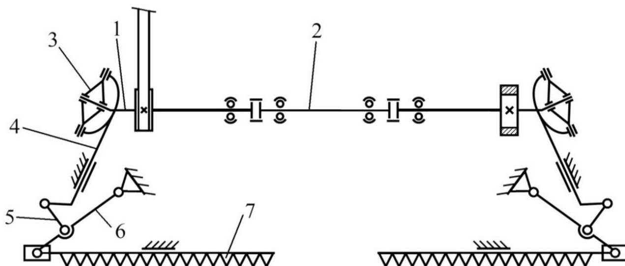
Рисунок 1 – Схема привода с механизмами «качающаяся шайба»
