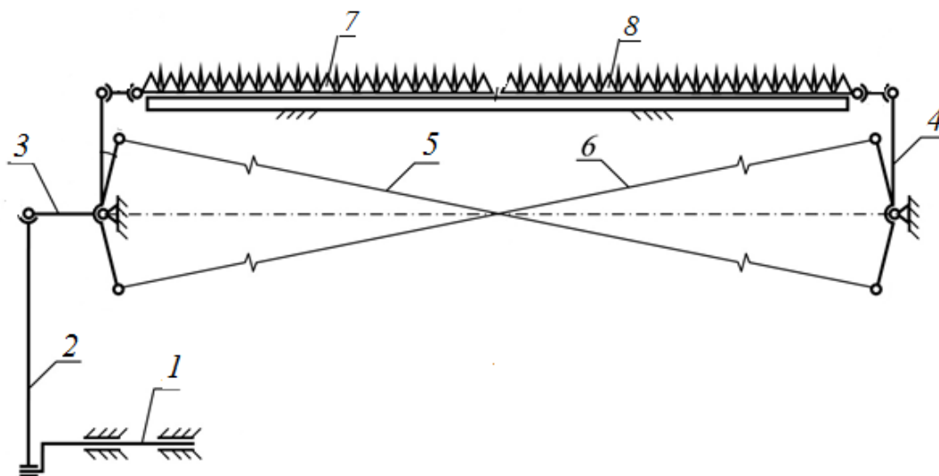
Рисунок 3 – Схема кривошипно-коромыслового механизма двухножевого режущего аппарата с гибкими тягами
