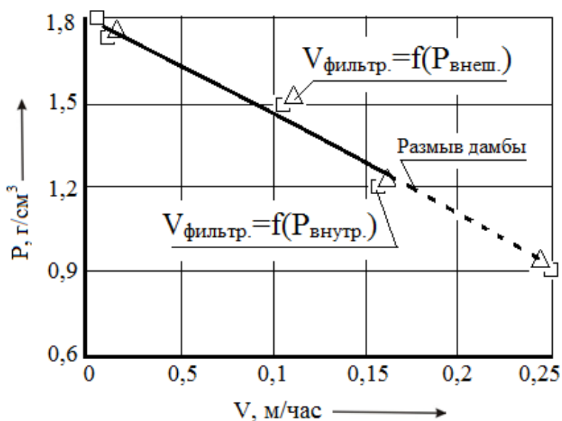
Рисунок 3 – Графики зависимости: V_{\text{филтр.}} = f(P_{\text{внеш.}}) ; V_{\text{филтр.}} = f(P_{\text{внутр.}})
