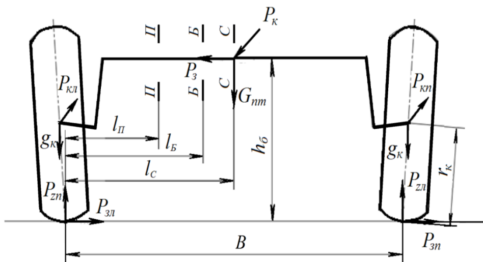
Рисунок 2 – Расчетная схема реверсивного переднего моста
