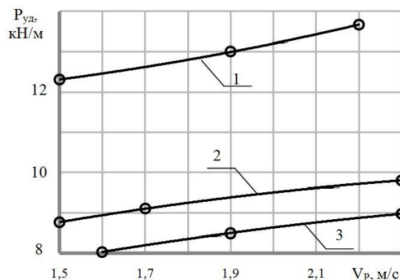
Рисунок 6 – Влияние скорости движения V_p на тяговое сопротивление плоскорежущего рабочего органа P_T
