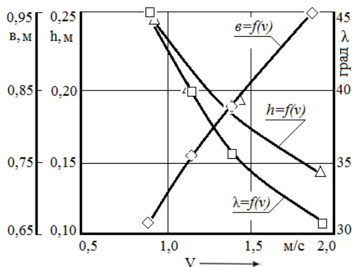
Рисунок 2 – Графики зависимости: h=f(v) ; \epsilon=f(v) и \lambda=f(v)
