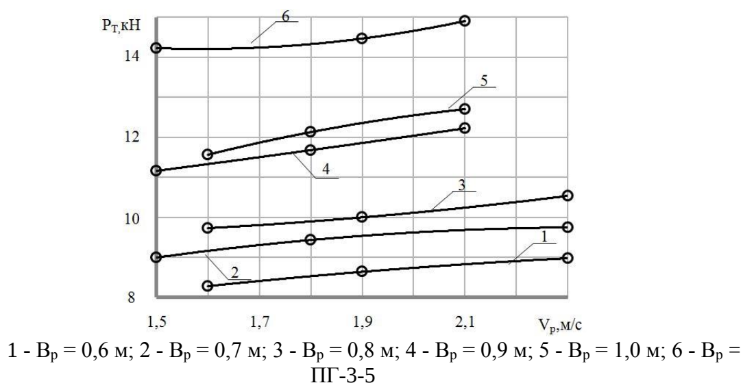
Рисунок 5 – Влияние рабочей скорости движения V_p на тяговое сопротивление плоскорежущих рабочих органов P_T
