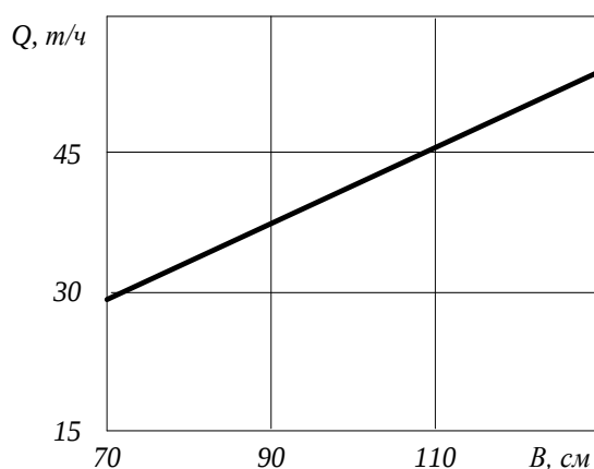
Рисунок 2 – Зависимость производительности пневмосепаратора Q от ширины воздушного канала B
