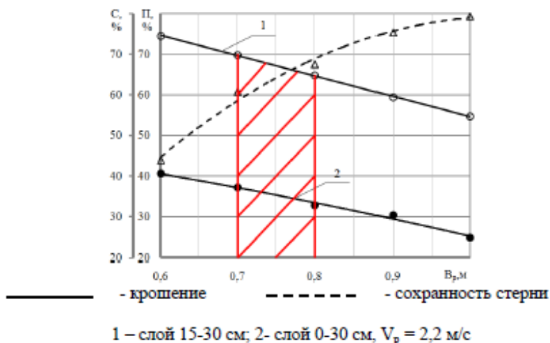
Рисунок 4 – Влияние ширины захвата рабочего органа V_r на крошение почвенного слоя \Pi и сохранность стерни на поверхности поля C
