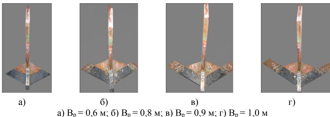
Рисунок 2 – Варианты плоскорежущих рабочих органов
