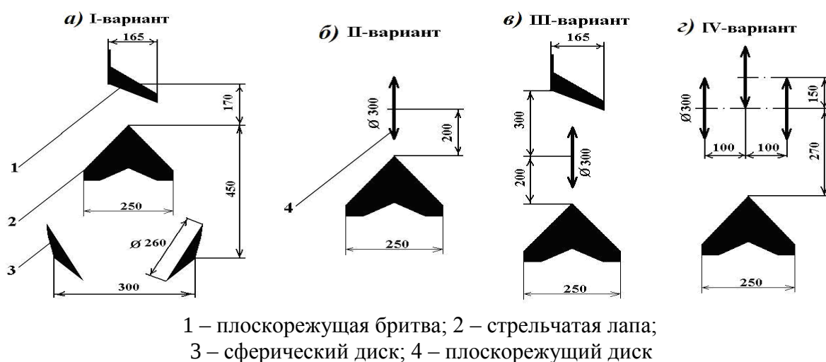
Рисунок 2 – Схемы размещения рабочих органов для минимальной обработки почвы
