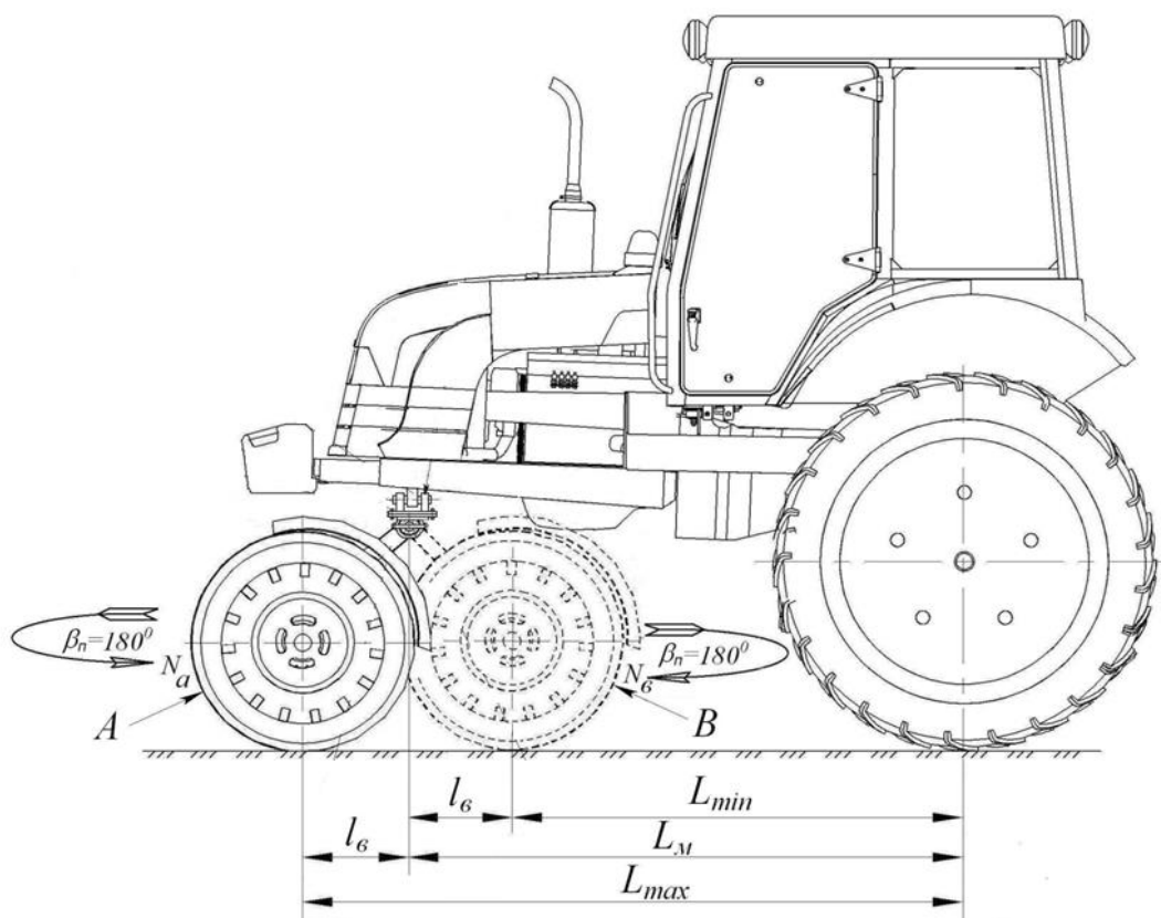
Рисунок 1 – Универсально-пропашной трактор, снабженный реверсивным передним мостом
