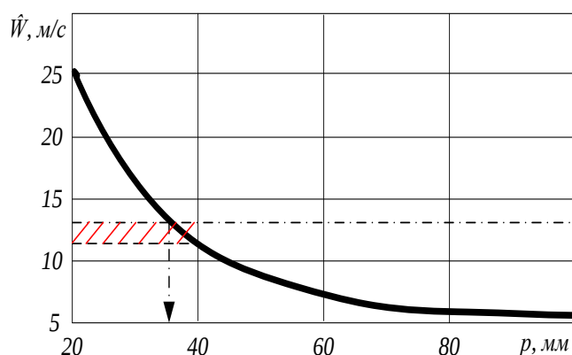
Рисунок 4 - Зависимость скорости воздушного потока W от размера калибра сопла p
